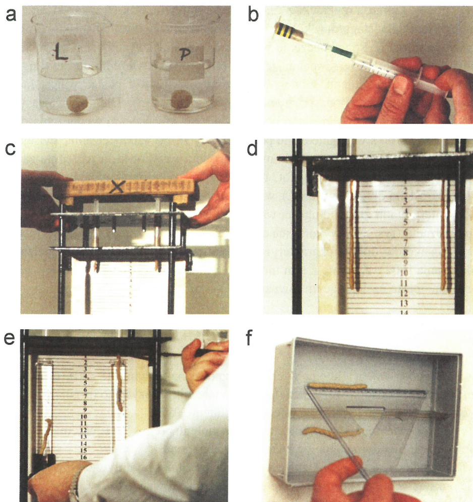
Fot. 1. Etapy przeprowadzania testów wytlaczania i pelzania walca glutenu mokrego: (a) próbki glutenu przygotowane do badań, (b) umieszczenie glutenu w strzykawce, (c) wytłaczanie glutenu i formowanie walca, (d) pelzanie walca glutenu pod własnym ciężarem i odczyt zmian jego długości, (e) koniec etapu pelzania; odcięcie i zanurzenie walca glutenu w solance, (f) etap odprężania, przy końcu którego odczytuje się długość walca
