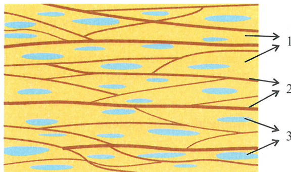
Rys. 5. Proponowany model struktury glutenu świeżo wymytego: 1 – gliadyny, 2 – gluteniny, frakcje 1 i 2 zawierają wodę związaną, 3 – woda niezwiązana
