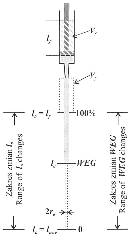
Rys. 8. Ilustracja zależności wskaźnika elastyczności glutenu (WEG) od długości wytłoczonego walca glutenu ( l_0 ); l_f – skok tłoka, V_f – objętość wytłoczonego glutenu, r_c – promień otworu wylotowego strzykawki, l_{max} = (V_f / \pi r_c^2)
