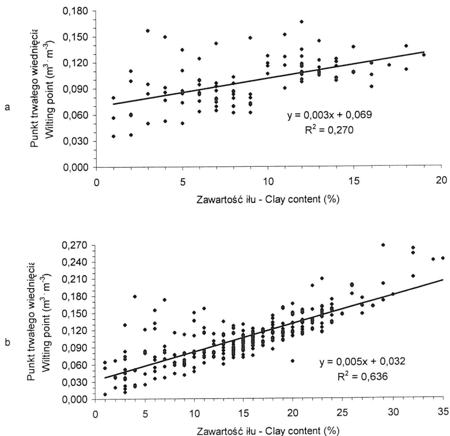
Rys. 11. Zależność pojemności wodnej w punkcie trwałego wędnięcia od zawartości iłu: a) w poziomie Ap, b) w poziomach podpowierzchniowych
