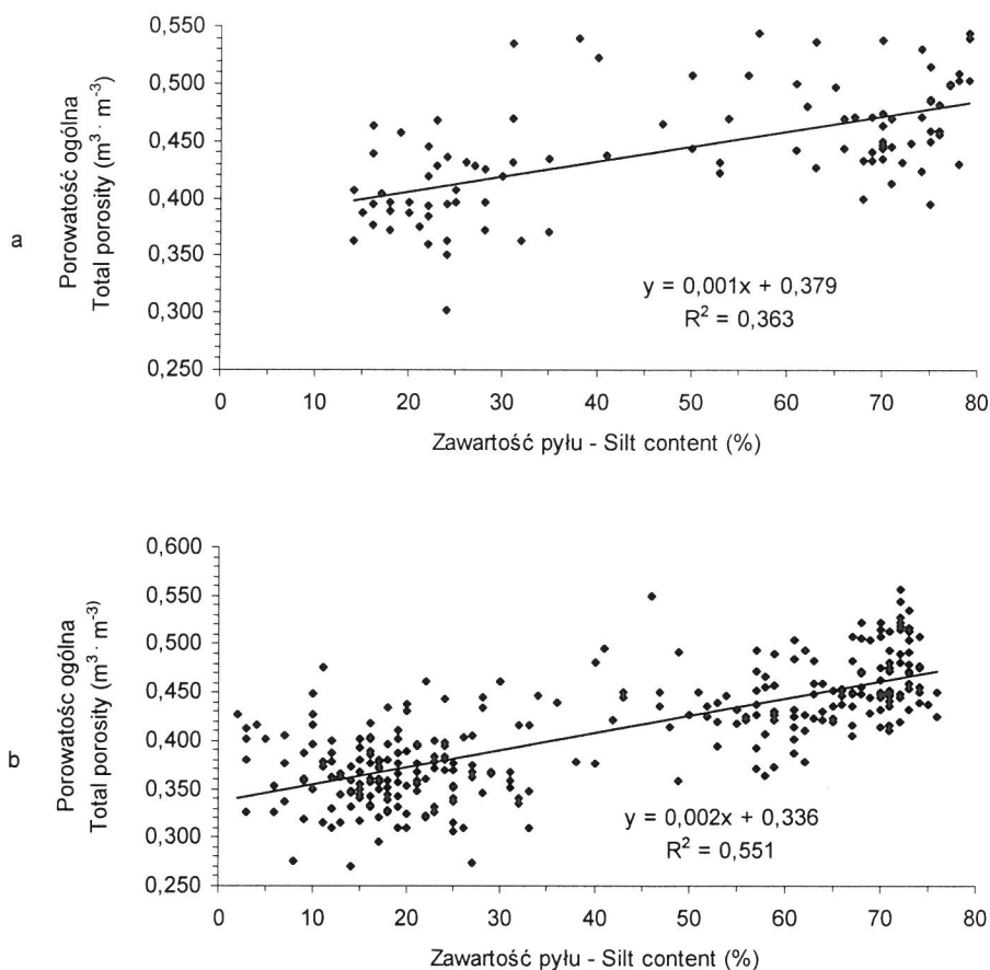
Rys. 8. Zależność porowatości ogólnej od zawartości pyłu: a) w poziomie Ap, b) w poziomach podpowierzchniowych
