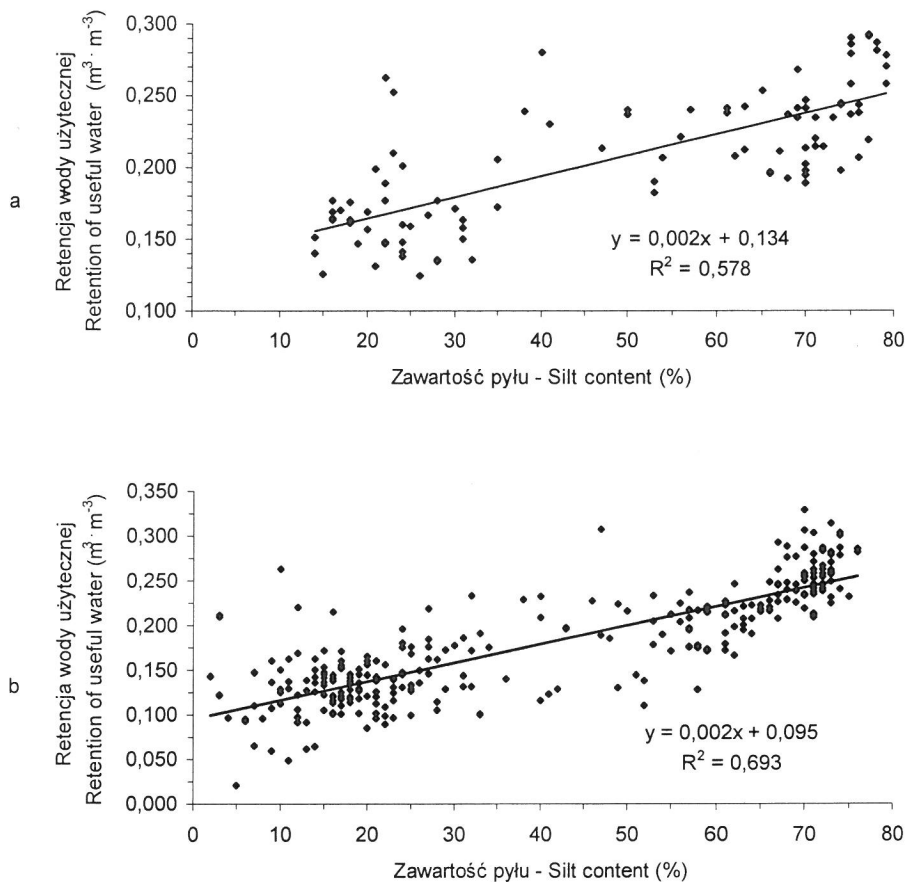
Rys. 14. Zależność retencji wody użytecznej od zawartości pyłu: a) w poziomie Ap, b) w poziomach podpowierzchniowych
