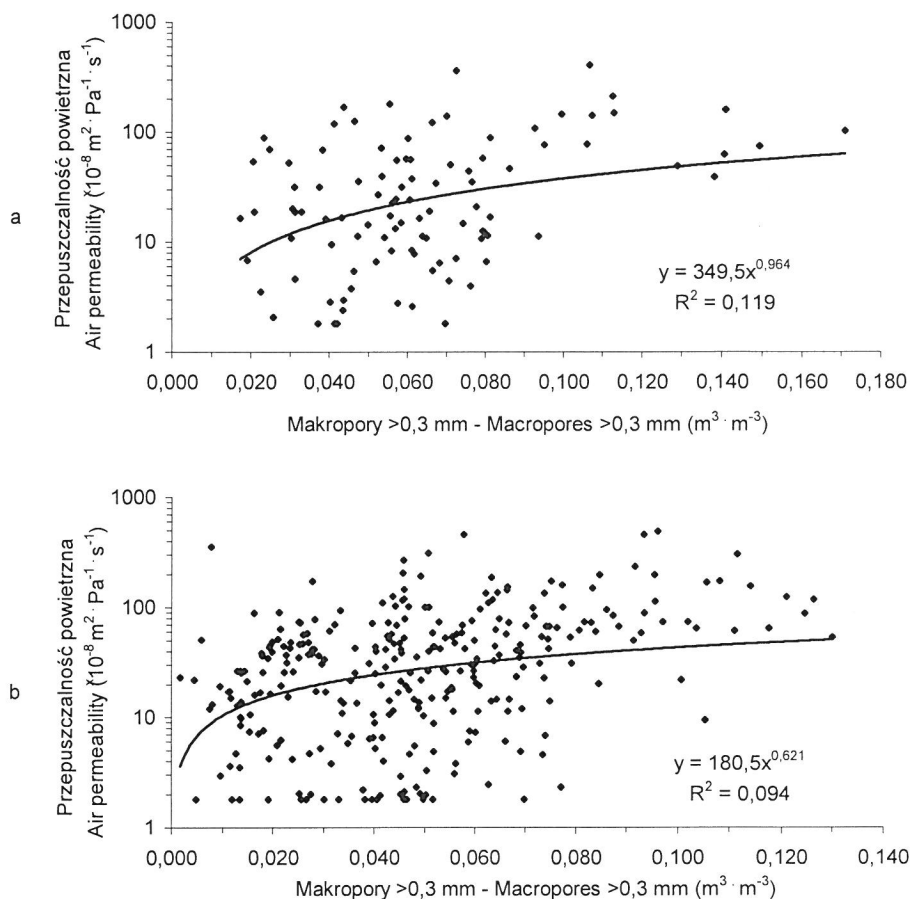
Rys. 19. Zależność przepuszczalności powietrznej (–15,5 kPa) od zawartości makroporów >0,3 mm: a) w poziomie Ap, b) w poziomach podpowierzchniowych
