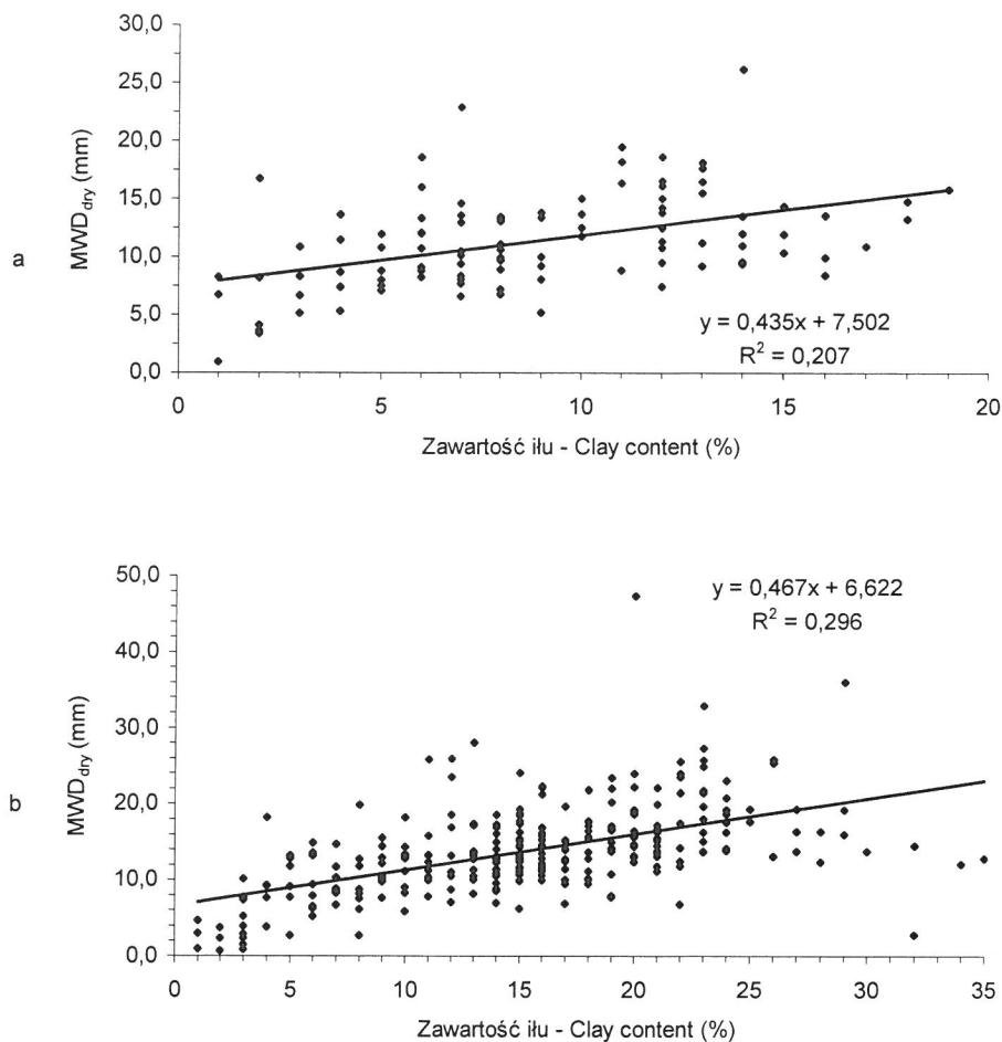
Rys. 3. Zależność średniej ważonej średnicy powietrznie suchych agregatów ( MWD_{dry} ) od zawartości ilu: a) w poziomie Ap, b) w poziomach podpowierzchniowych
