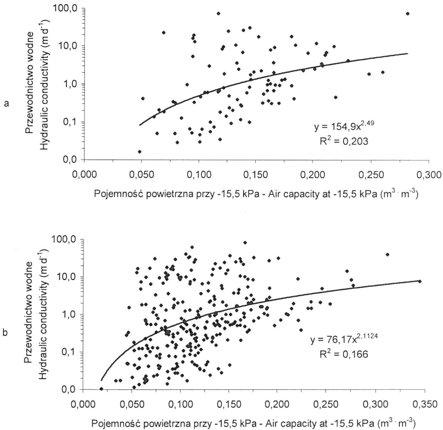
Rys. 16. Zależność przewodnictwa wodnego nasyconego od pojemności powietrznej ( -15,5\ \text{kPa} ): a) w poziomie Ap, b) w poziomach podpowierzchniowych
