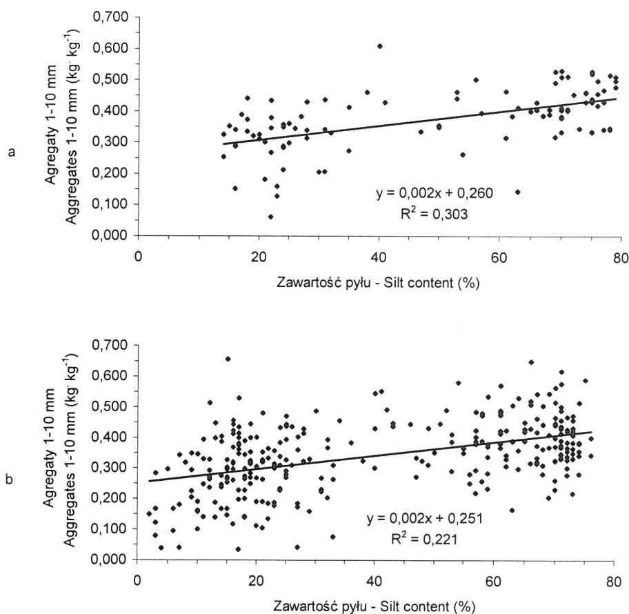
Rys. 2. Zależność zawartości powietrznie suchych agregatów 1-10 mm od zawartości pyłu: a) w poziomie Ap, b) w poziomach podpowierzchniowych
