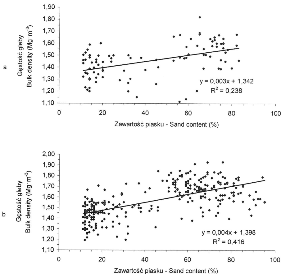
Rys. 7. Zależność gęstości gleby od zawartości piasku: a) w poziomie Ap, b) w poziomach podpowierzchniowych
