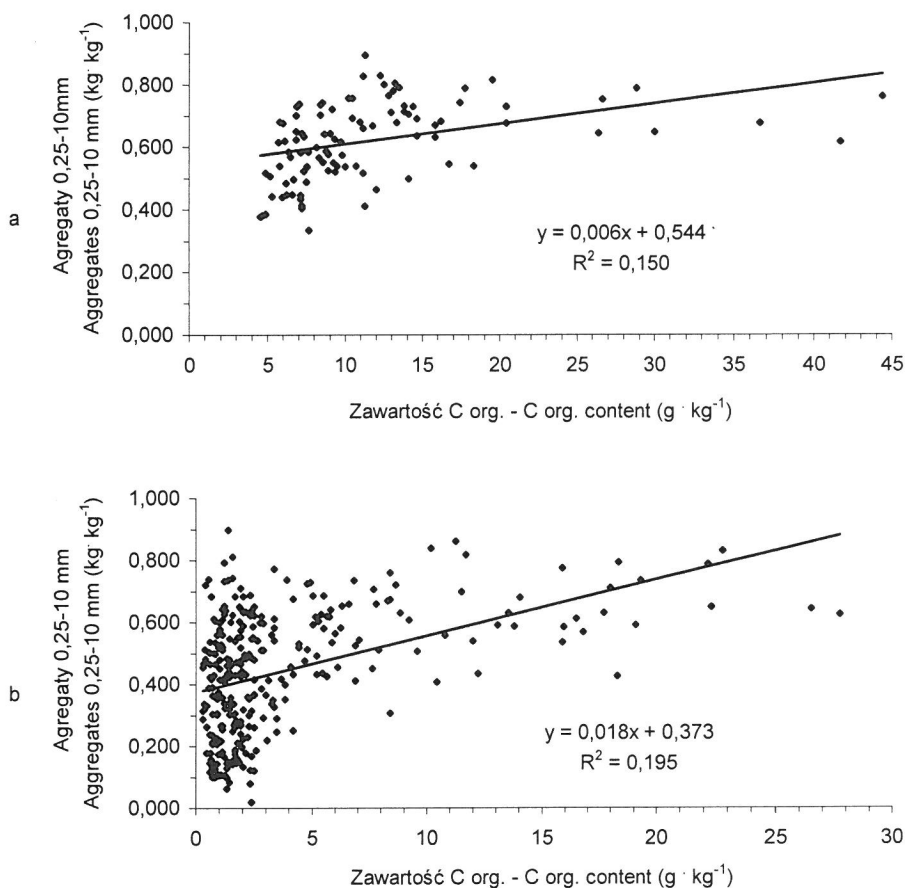
Rys. 4. Zależność zawartości wodoodpornych agregatów 0,25-10 mm od zawartości C org.: a) w poziomie Ap, b) w poziomach podpowierzchniowych
