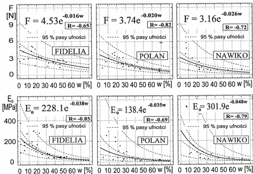
Rys. 3. Siła F zniszczenia podczas rozciągania okrywy nasion grochu odm. Fidelia i soi odm. Polan i Nawiko oraz moduł sprężystości E_0 wyznaczony w zakresie niewielkiej deformacji.
