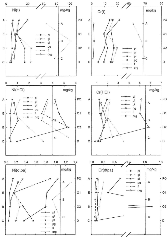
Rys. 4. Zawartość różnych form Ni i Cr (mg/kg): pl – piaski luźne i słabogliniaste (A, E, B, C), pg – piaski gliniaste (A, B, C), gl – gliny (A, E, B, C), pł – utwory pyłowe (A, E, B, C), fl – gleby utworzone z fliszu karpackiego (A, B, C), org – torfy różnego pochodzenia (PO, O1, O2, D).
