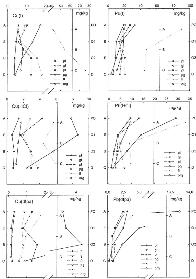
Rys. 2. Zawartość różnych form Cu i Pb (mg/kg): pl – piaski luźne i słabogliniaste (A, E, B, C), pg – piaski gliniaste (A, B, C), gl – gliny (A, E, B, C), pł – utwory pyłowe (A, E, B, C), fl – gleby wytworzone z fliszu karpackiego (A, B, C), org – torfy różnego pochodzenia (PO, O1, O2, D).
