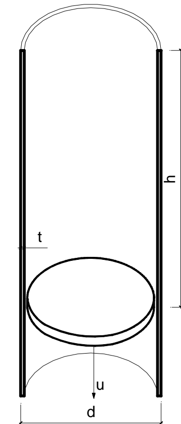
Rys. 1. Schemat przepływu kontrolowanego materiału sypkiego w silosie Fig. 1. Controlled flow of bulk solid in silo (schematically)
