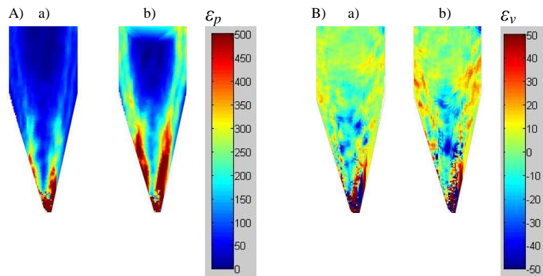
Rys. 5. Zmiana odkształceń postaciowych \varepsilon_p (A) oraz objętościowych \varepsilon_v (B) w luźnym piasku średnioziarnistym d_{50} = 0,8 \text{ mm} w silosie ze ścianami bardzo szorstkimi i przepływem masowym: a) 1 s, b) 5 s (wypływ grawitacyjny)
